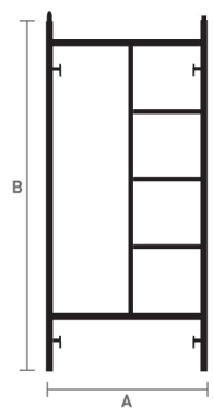
LATERAL DE ANDAIME MARCO DE ANDAMIO LATÉRAL D'ÉCHAFAUDAGE SIDE OF SCAFFOLD SCAFFOLDS SEITE E.04010.4211
