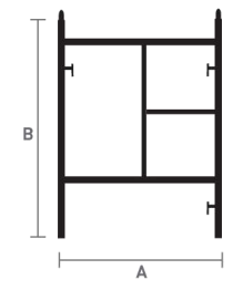
LATERAL DE ANDAIME 1000mm MARCO DE ANDAMIO 1000mm LATÉRAL D'ÉCHAFAUDAGE 1000mm SIDE OF SCAFFOLD 1000mm SCAFFOLDS SEITE 1000mm E.04010.4100
