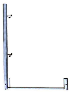
1000 x Ø48 x 2,5 mm - GALVA TUBO TERMINAL GUARDA COSTAS TUBO GUARDA-ESPALDAS TUBE TERMINALE POUR GARDE CORPS TUBE TERMINAL GUARD BACK TERMINAL ROHR LEIBGARDE E.75540.1215
