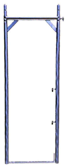
2000 x 750 mm Ø48 x 2,6 mm - GALVA
