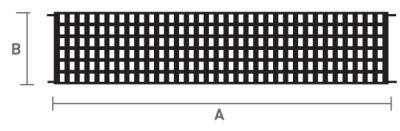
PRANCHA METÁLICA 300 PT PLATAFORMA 300 PT PLANCHER MÉTALLIQUE 300 PT METALIC BOARD 300 PT METALLPLANKE 300 PT E.04010.4230 PRANCHA METÁLICA 400 PT PLATAFORMA 400 PT PLANCHER MÉTALLIQUE 400 PT METALIC BOARD 400 PT METALLPLANKE 400 PT E.04010.4240
