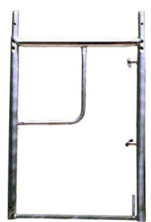
2000 x 750 mm Ø48 x 2,6 mm - GALVA
